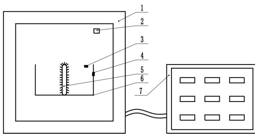
1—箱体；2—湿度控制系统；3—喷淋系统；4—黑标准（板）温度控制系统； 5—氙灯；6—试样架；7—试验设备总控制系统。
