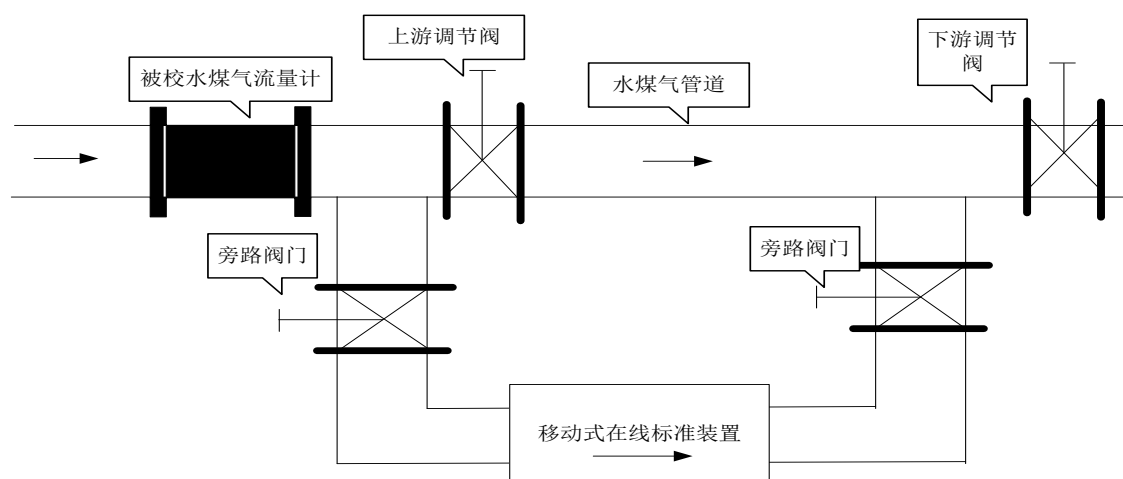
图 1 串联移动式装置校准图
