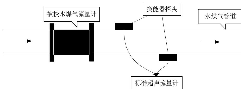
图 2 标准表法（外夹式超声流量计）工作原理图
